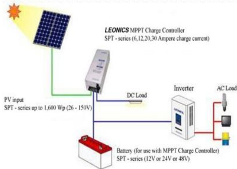
Figure1: MPPT
